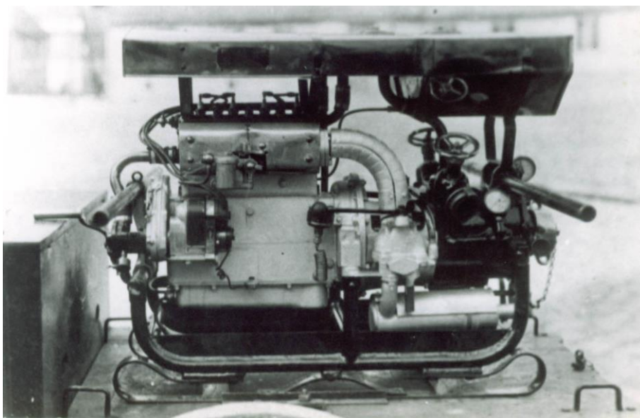
1926.gadā iegādātā biedrības pirmā motoršļirce.
